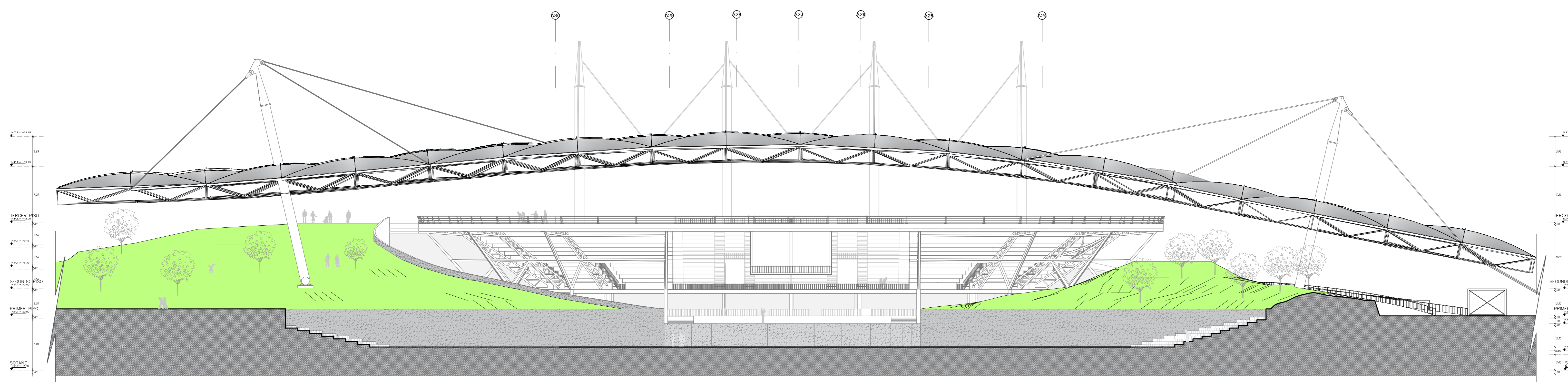
ELEVACION 2 – LATERAL 1
