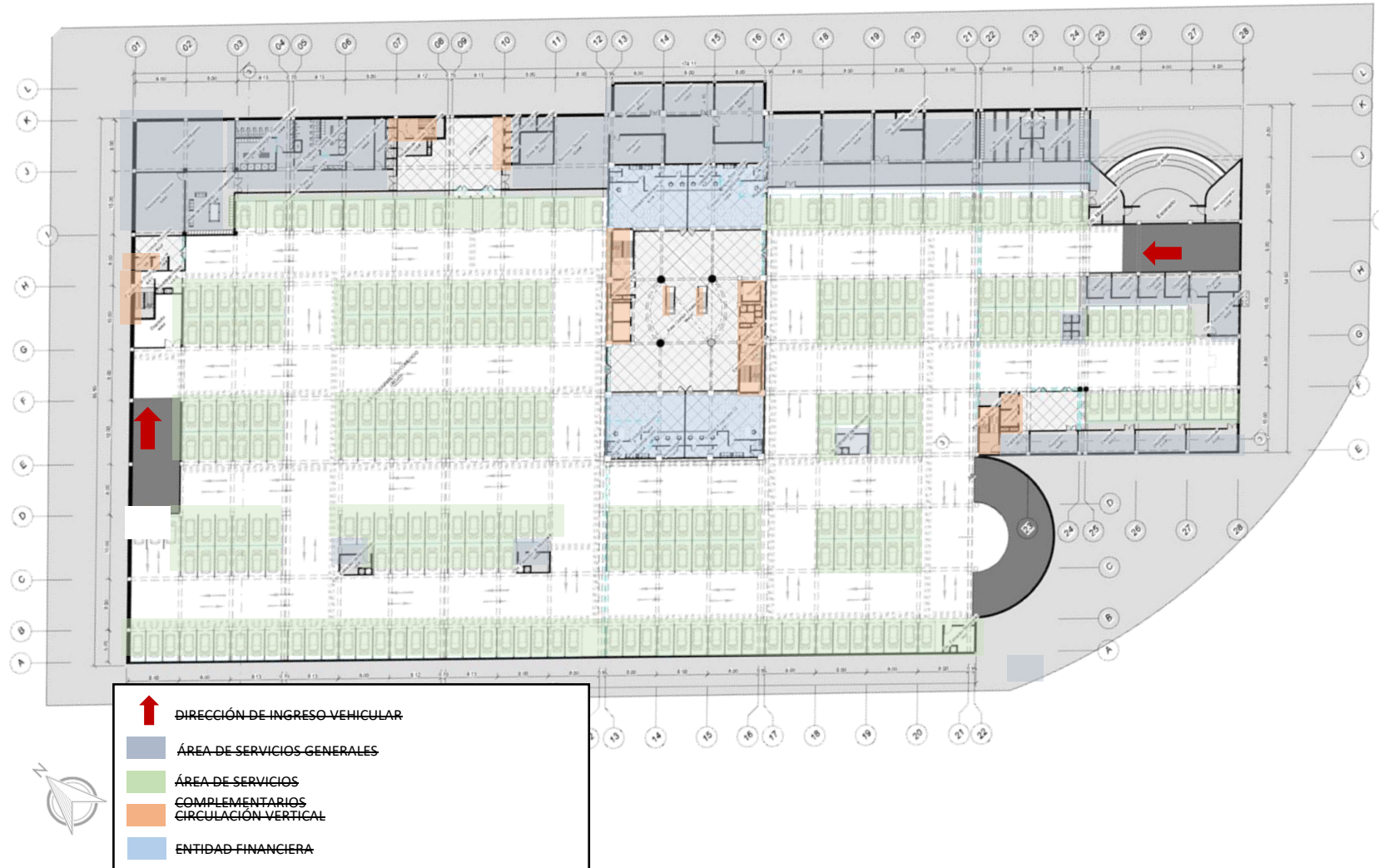
Plano Sótano 01
