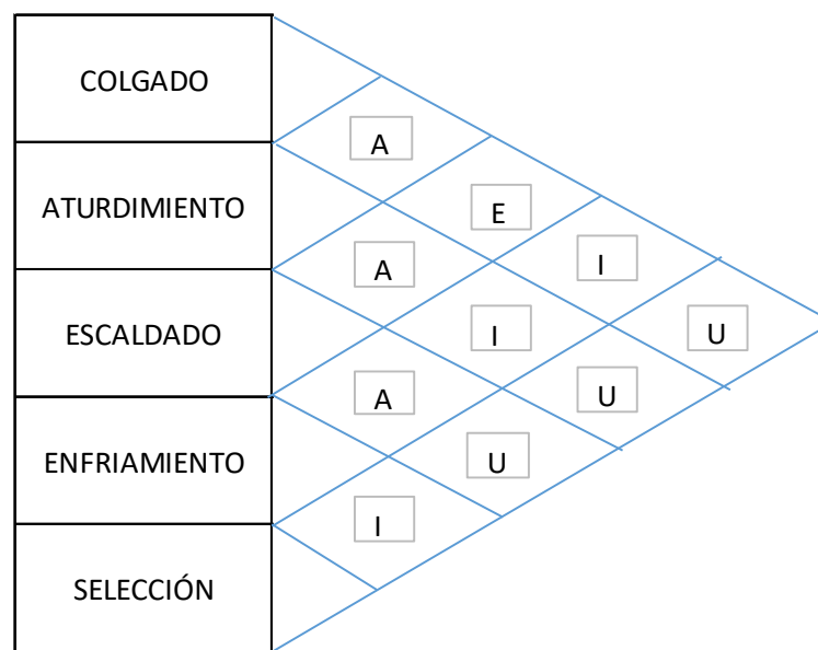
Figura 26: Diagrama relacional de actividades del área de beneficiado Elaboración: Propia
