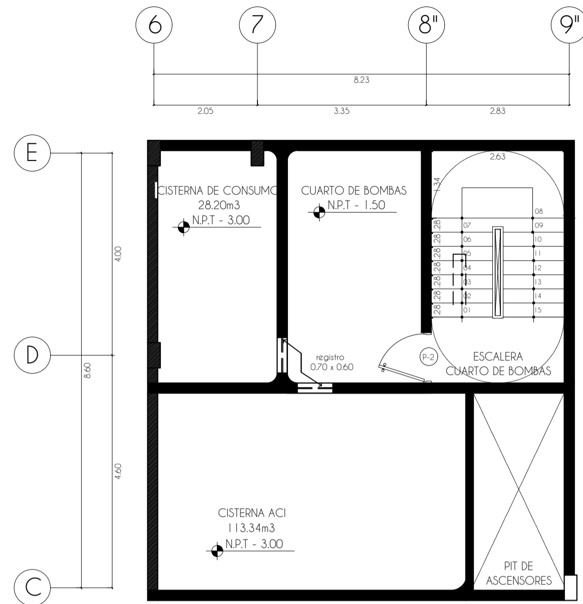
PLANTA DE CUARTO DE BOMBAS - TIPO A
