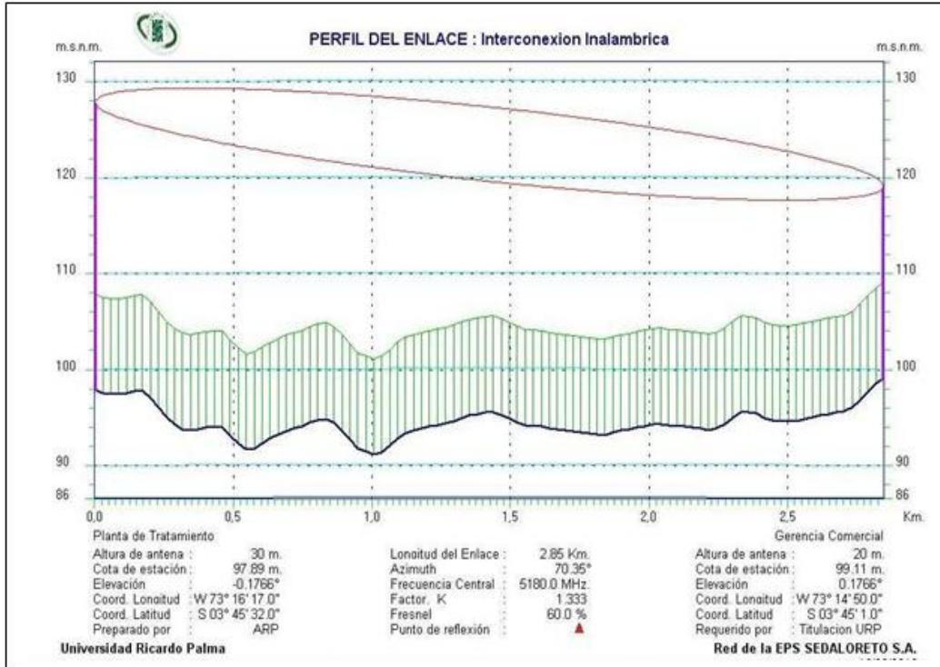
Figura 3.10: Perfil del Enlace
