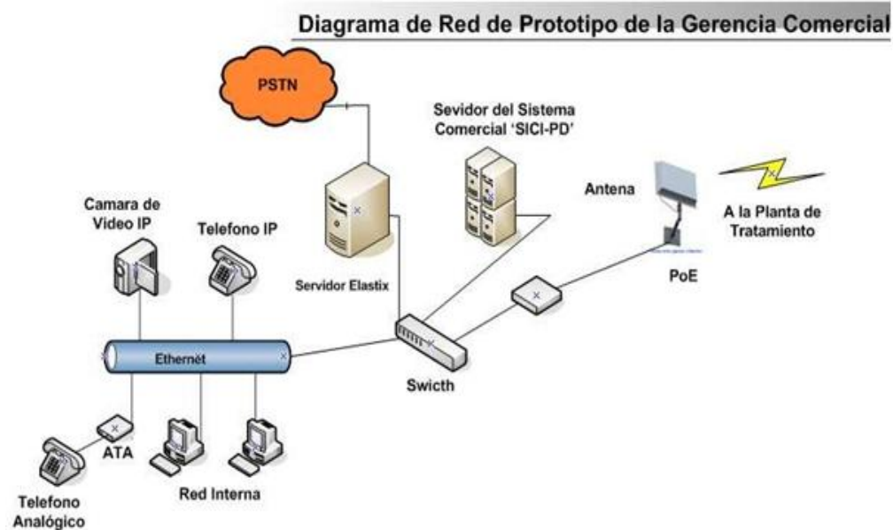
Figura 3.20: Se muestra el Prototipo de Red de la Gerencia Comercial
