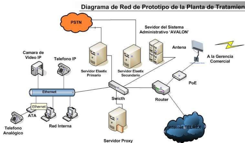
Figura 3.19: Se muestra el Prototipo de Red de la Planta de Tratamiento
