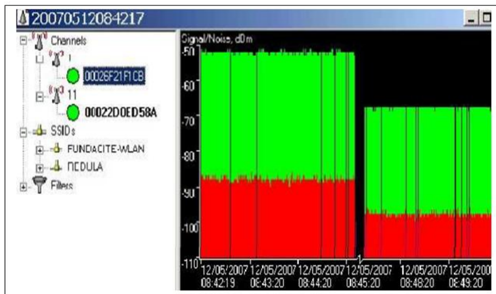
Figura 3.4: Señal y Ruido con y sin amplificar.
