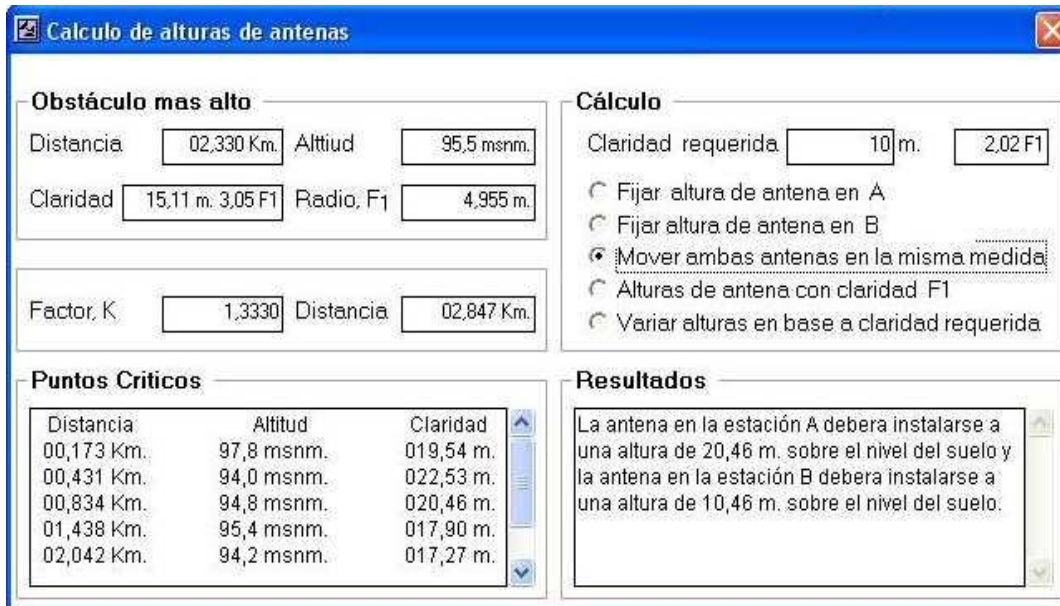
Figura 3.11: Calculo de altura de las Antenas
