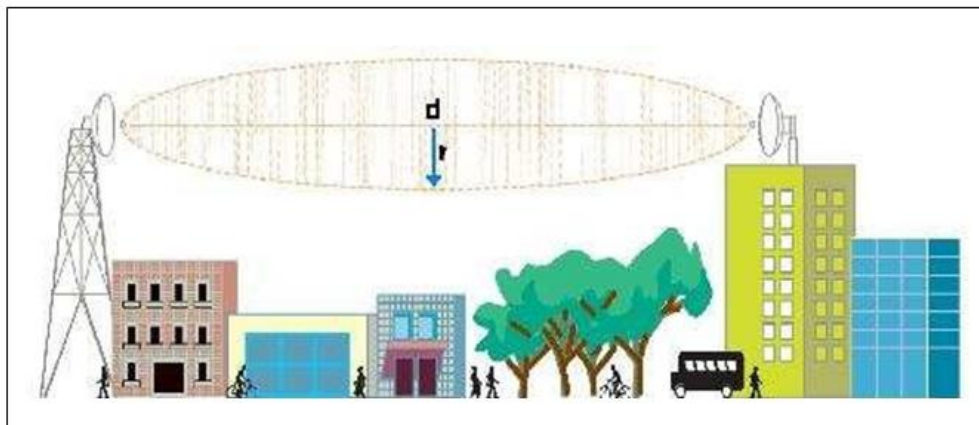
Figura 3.7: Zona de Fresnel
