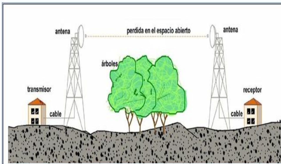
Figura 3.3: Trayectoria completa de transmisión entre el transmisor y el receptor Figura tomada de TRICALCAR | www.wilac.net/tricalcar – Versión final. Octubre 2007
