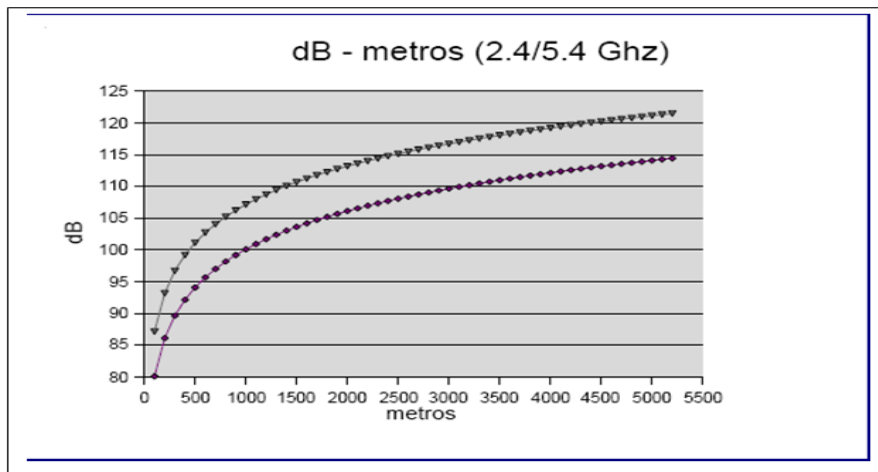
Figura 3.6: Pérdida en dB en función de la distancia en metros.
