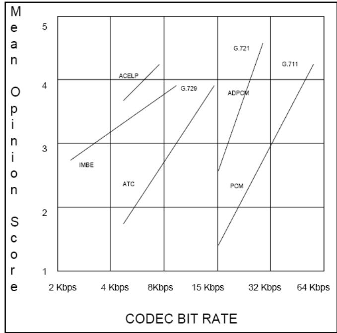
Figura 2.1: Comparación de la calidad de voz percibida (MOS) Grafico sacado de: CALIDAD DE LA VOZ:
