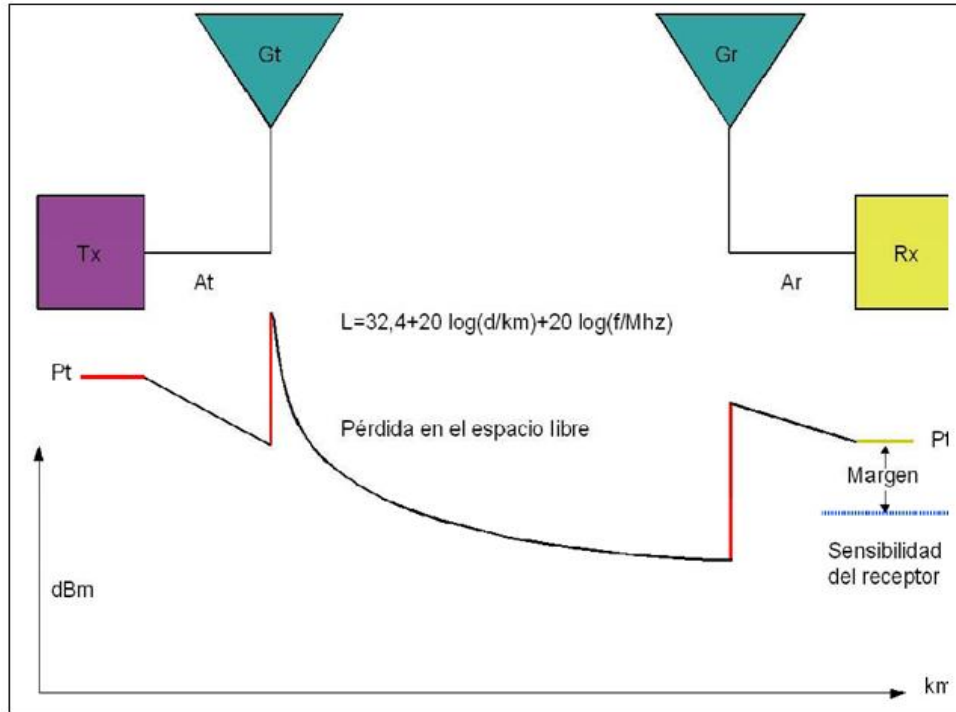
Figura 3.2: Potencia en dBm en función de la distancia para un radioenlace. Figura tomada de TRICALCAR | www.wilac.net/tricalcar – Versión final. Octubre 2007
